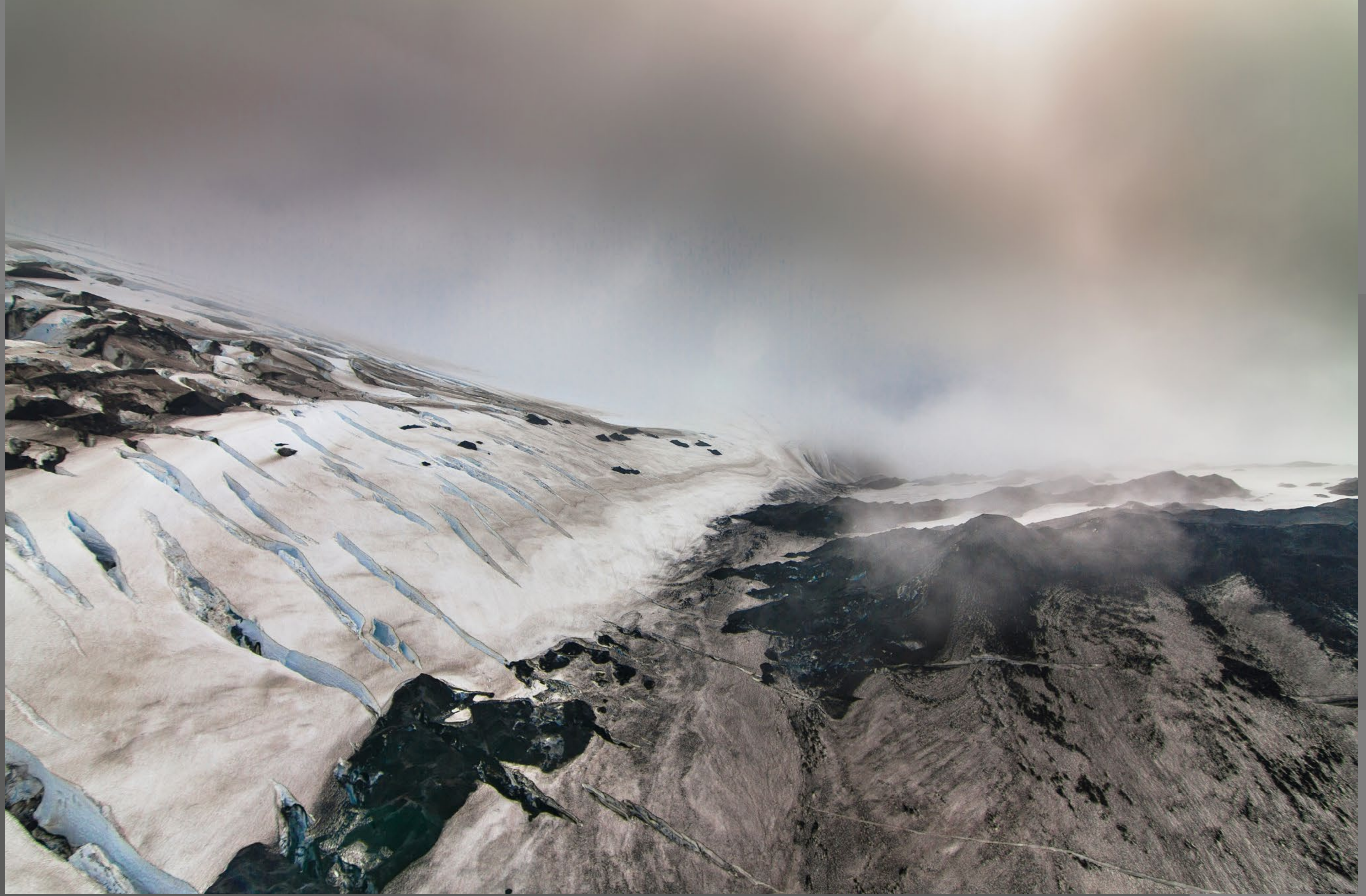
Eyjafjallajökull
