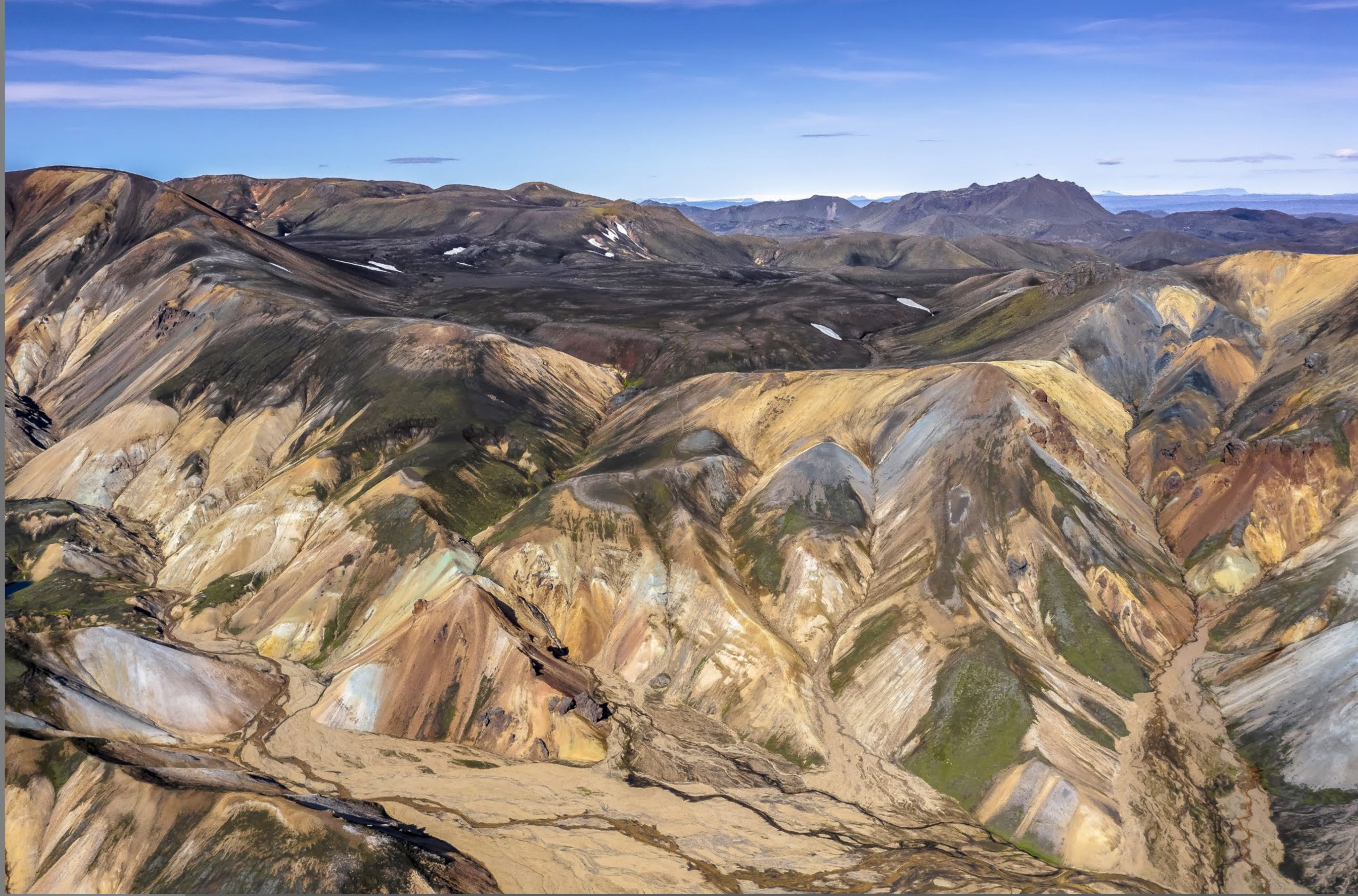
Landmannalaugar
